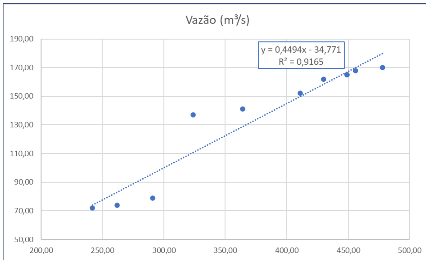
Gráfico Nível x Vazão
