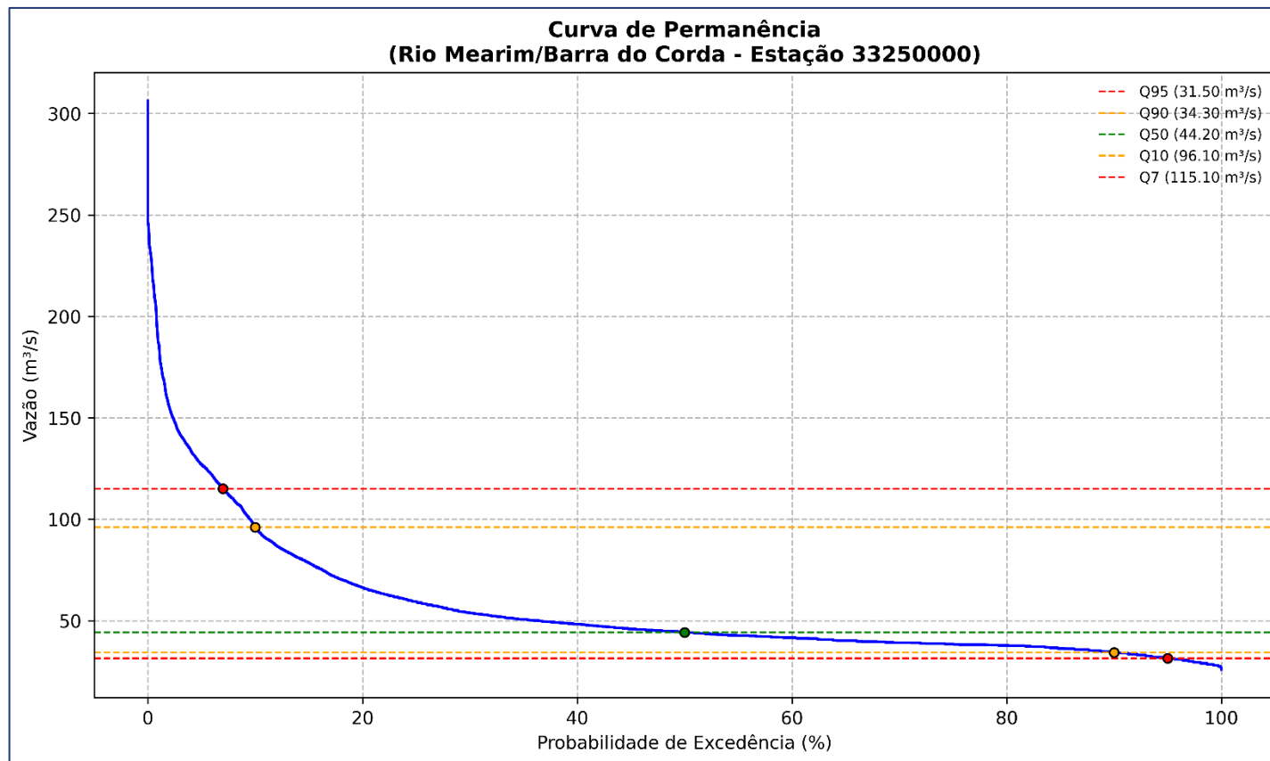
Gráfico da Curva de Permanência.
