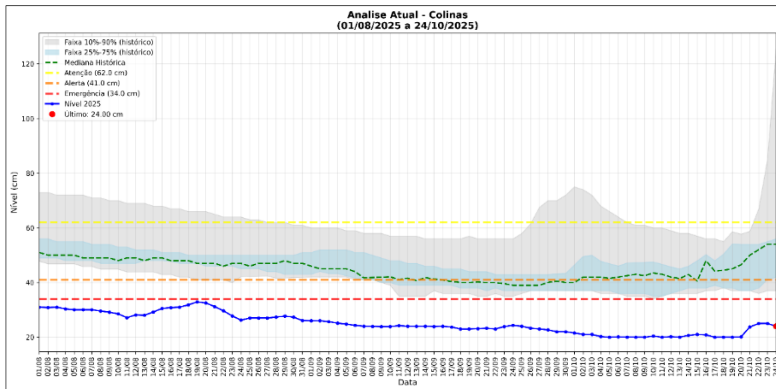
Serie Histórica da Estação Colinas, rio Itapecuru-Mirim
