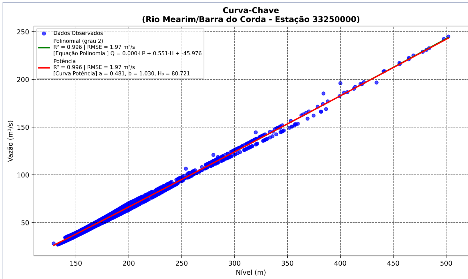
Curva-Chave da Estação de Barra do Corda
