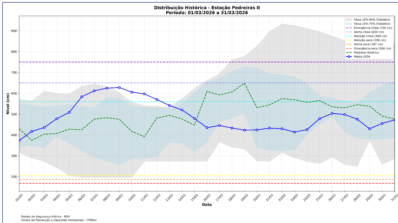
Histograma do rio Mearim em Pedreiras/MA
